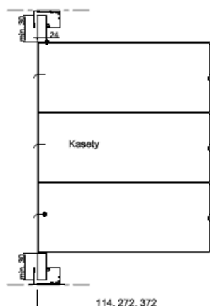
Schemat GRD(k) E – do profili PCV stałe drzwi, witryny PCV
